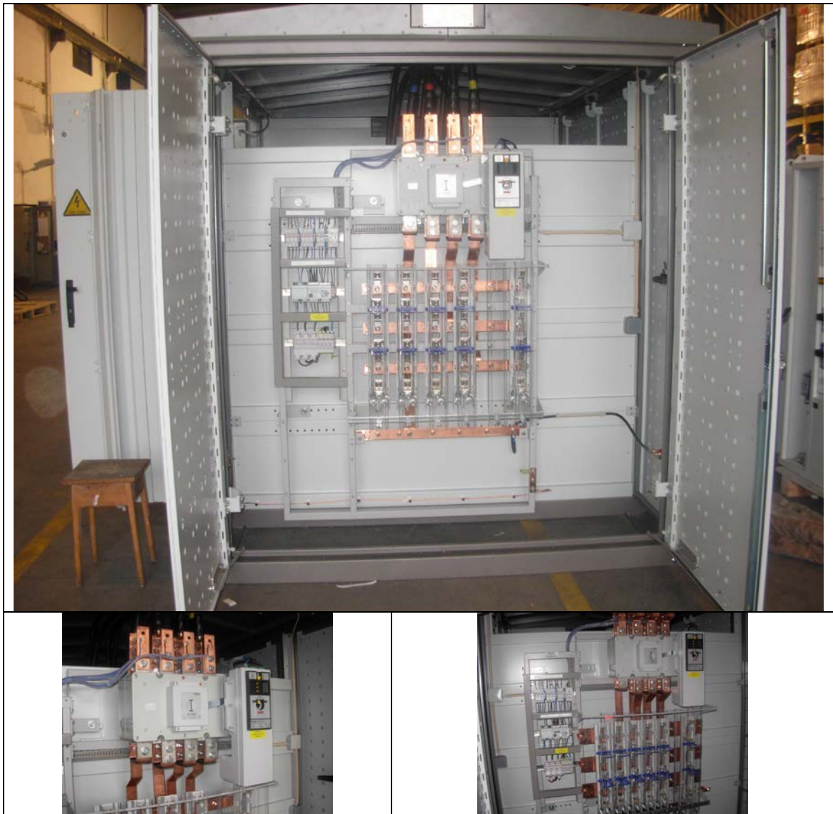
Quadro Aberto com Inversor Automático Rede/Grupo Montado em posto de transformação IBERKIT
